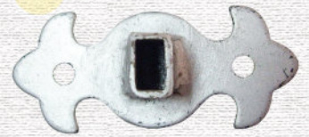
PE-01A 28x70x2mm. [5 x 10 mm.]
